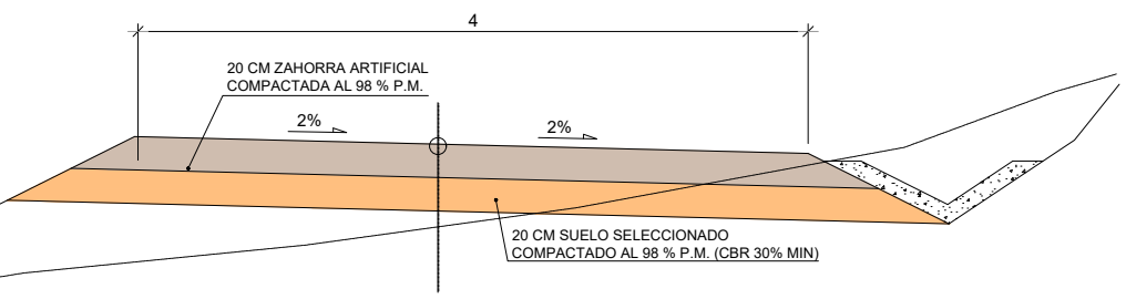
SECCION TIPO CAMINO INTERNO S:1/50
