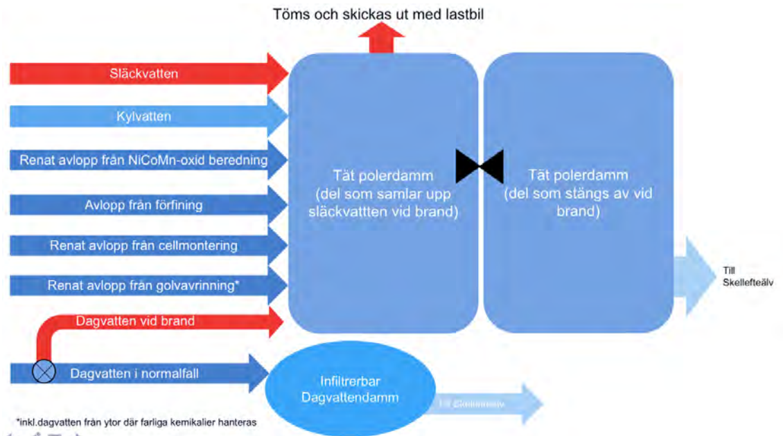
Figur 19. Schematisk bild som visar delflöden av renat vatten som leds vidare till Skellefteälven.
