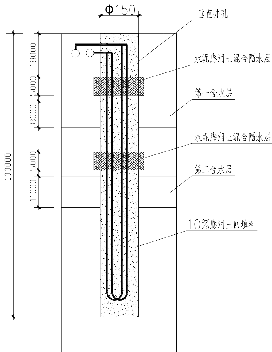
水泥隔水层示意图
