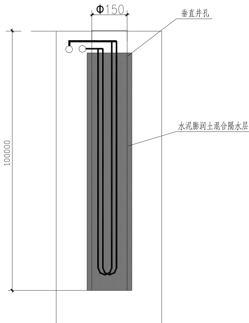
水泥隔水层示意图
