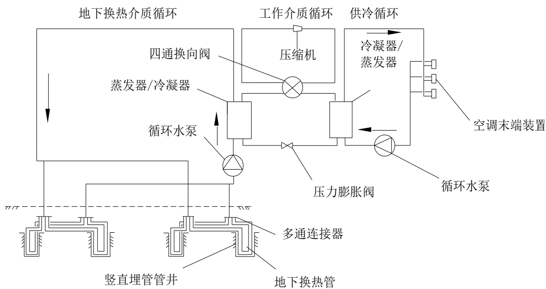
图 1 地源热泵冷热源空调系统原理图
