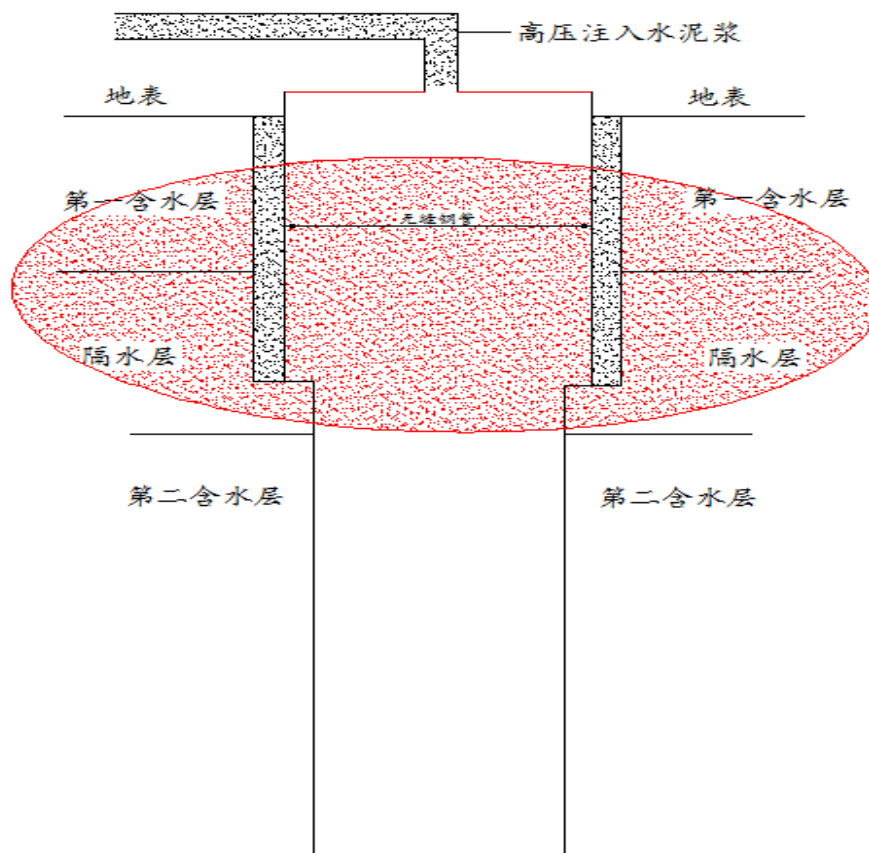
井口密封大样图
