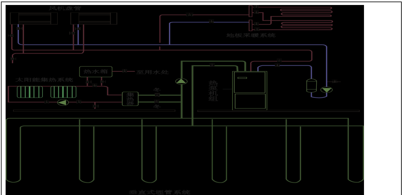
图2 太阳能-地源热泵复合系统原理图
