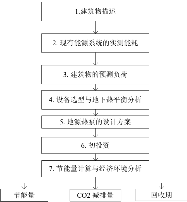
图 3 能源中心设计程序流程图
