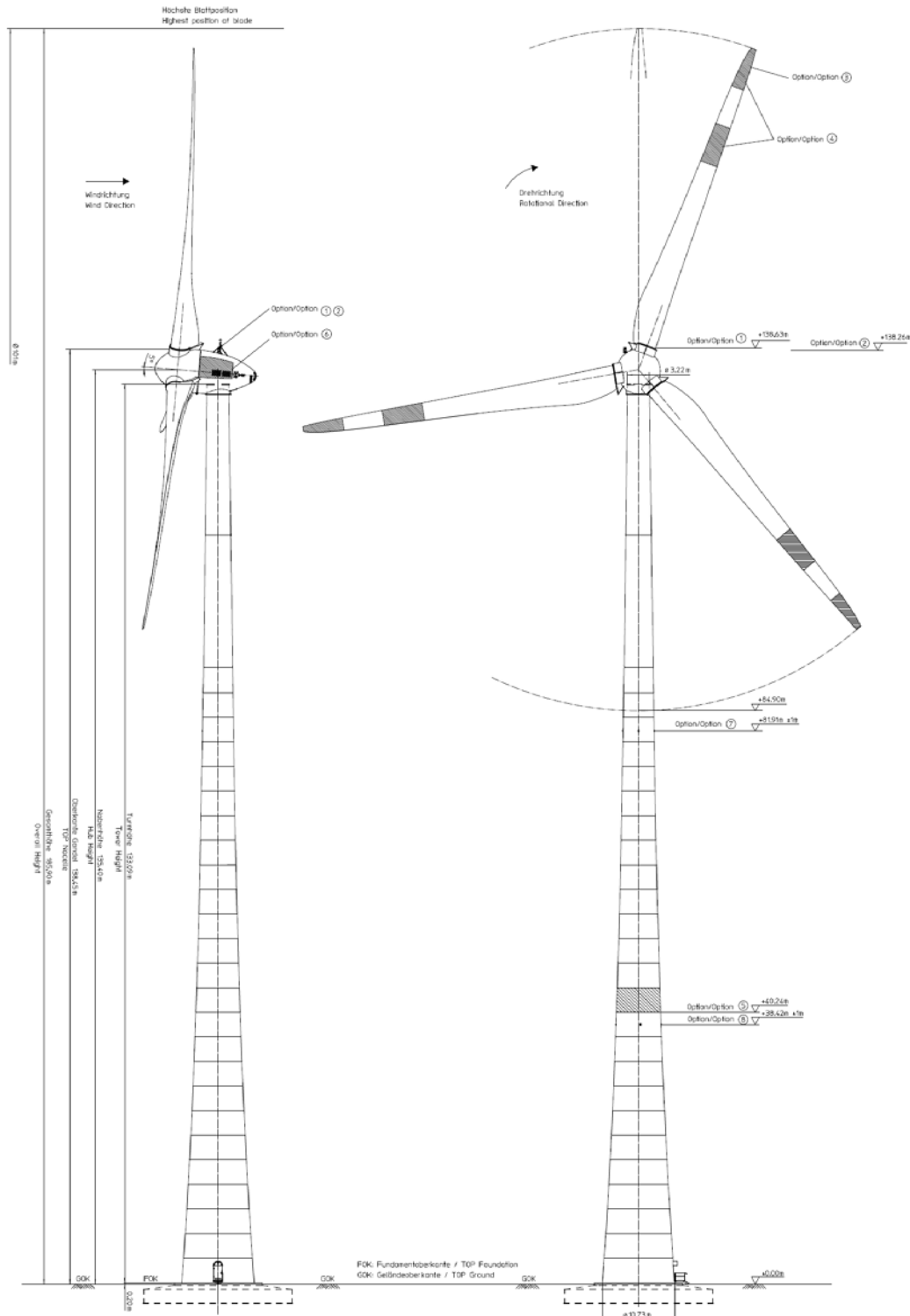
Abbildung 4: Ansichtsplan WKA Enercon E 101 mit 135,4 m Nabenhöhe, Quelle Fa. Enercon
