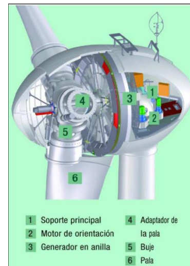
Imagen 1. Sección Góndola aerogenerador
