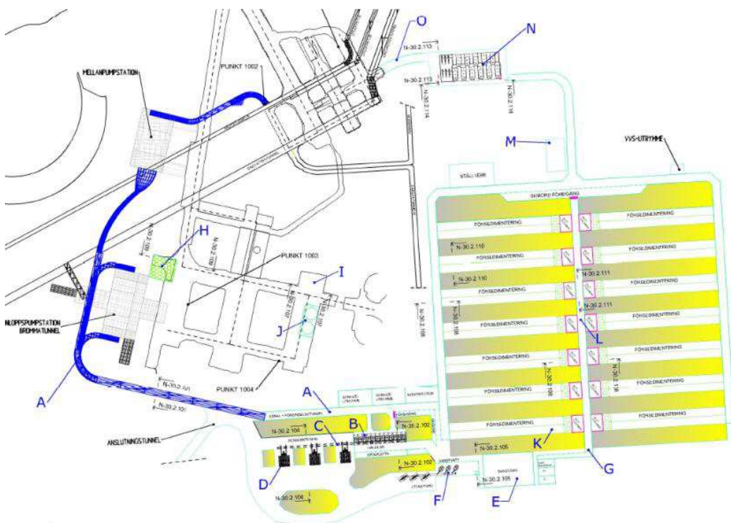
Figur 4-2: Layout av den utbyggda Sicklaanläggningen
