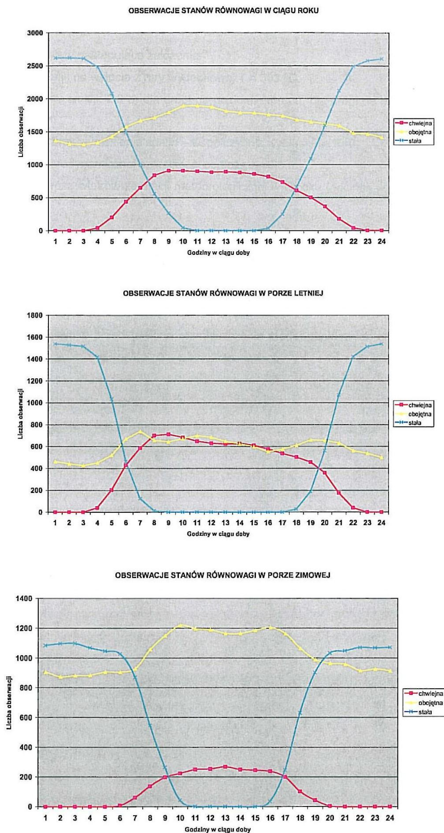
Rysunek 14.2.1 Stany równowagi (chwiejnej, obojętnej, stałej) występujących w ciągu roku, w porze letniej i porze zimowej w poszczególnych godzinach doby.
