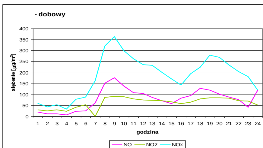
Rysunek 15.2.2. Dobowy przebieg stężeń NO 2 , NO i NO x na przykładowej stacji pomiarowej (emisja ze źródeł komunikacyjnych w Warszawie)
