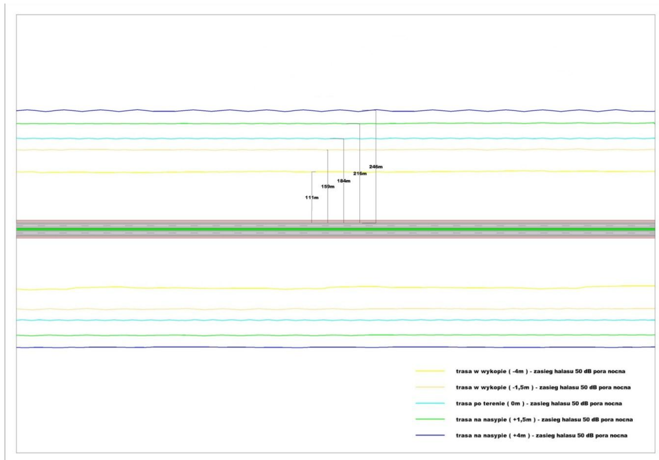
Rysunek 14.1.1 Wpływ zmiany niwelety trasy na zasięg hałasu – prognoza ruchu na rok 2015
