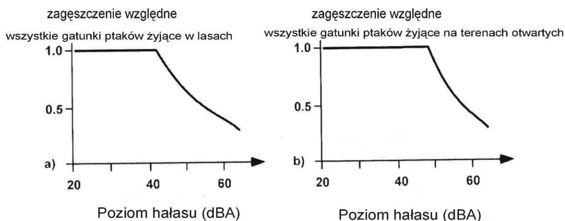
Rysunek 5.11.1 Wpływ poziomu hałasu na zagęszczenie względne gatunków ptaków leśnych i terenów otwartych
