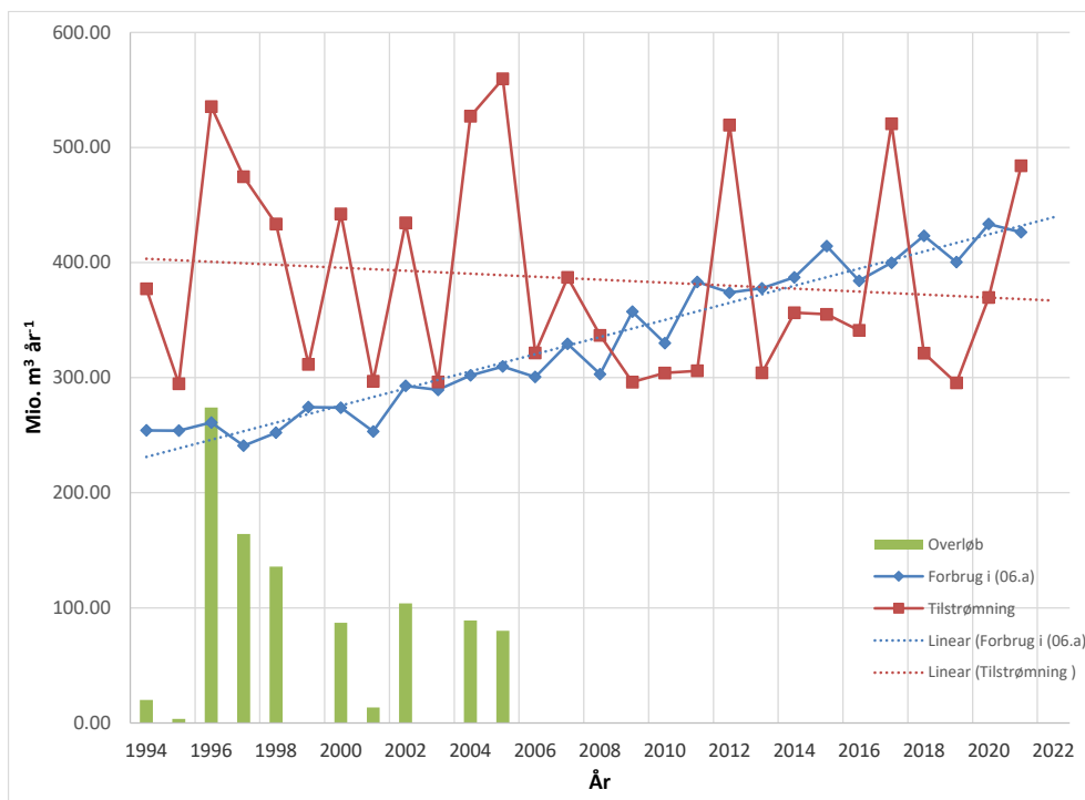
Figur 28: Oversigt over årlig tilstrømning, overløb og forbrug af produktionsvand (mio m³ år -1 ) i perioden 1994-2021 (data fra Nukissiorfiit).
