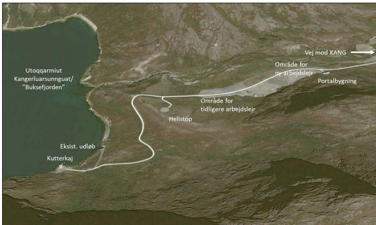
Figur 6: Infrastrukturanlæg m.m. i anlægsområdet ved Buksefjorden
