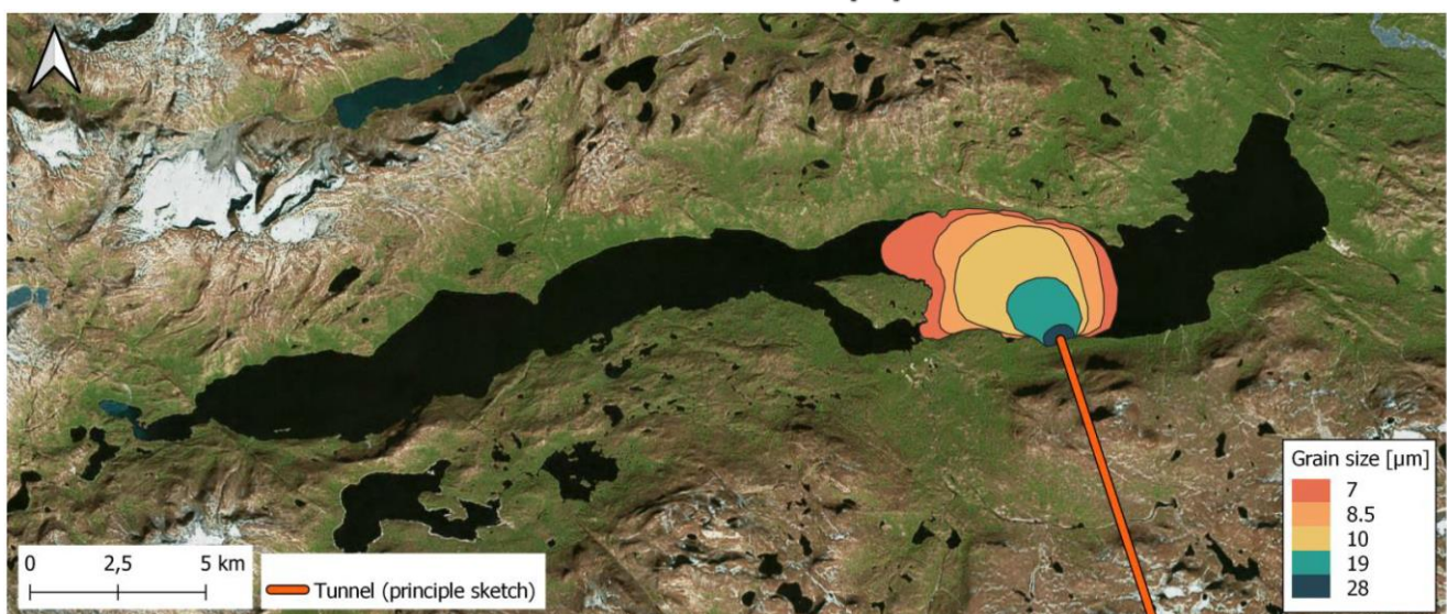
Figur 33: Modelberegninger som viser sedimentation af suspenderet materiale fra ISTA efter udledning i KANG (Niras, 2022a).
