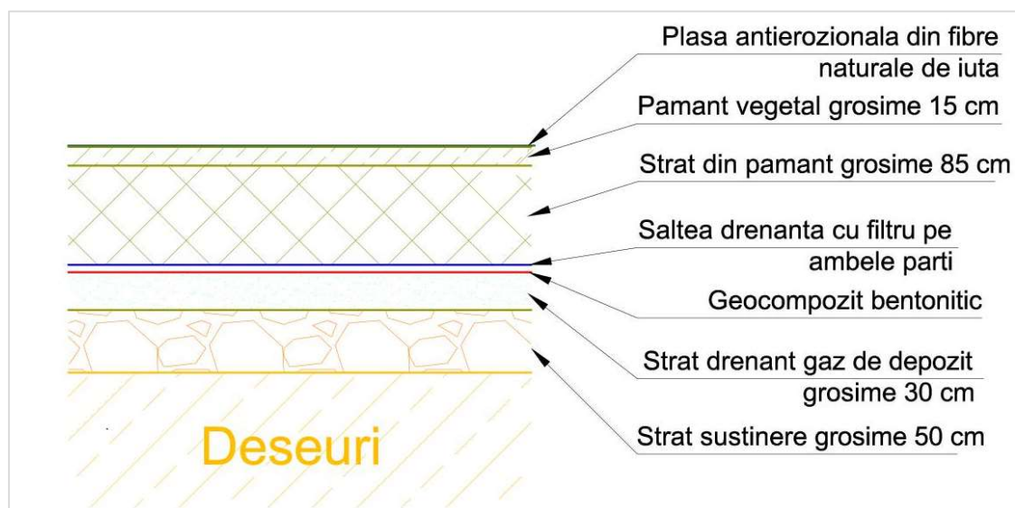
Figura 2-16: Sistemul de impermeabilizare al depozitului neconform Rateș - Tecuci
