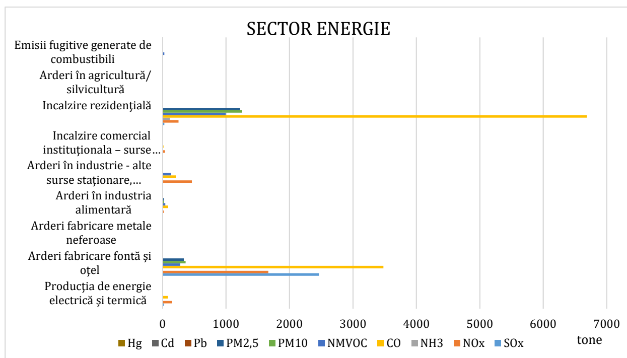
Figura 5-10: Emisiile de poluanți în atmosferă din sectoarele de activitate din energie
