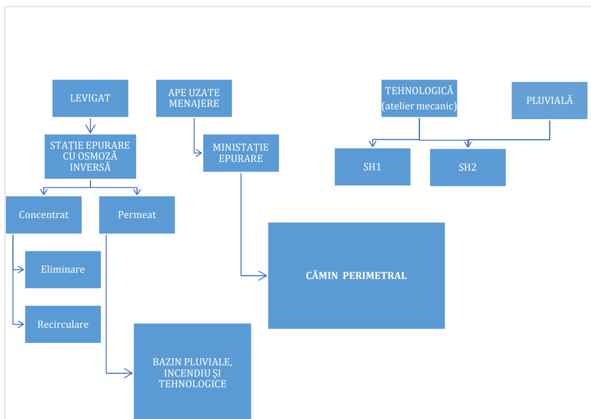
Figura 2-21: Traseul apelor evacuate și al levigatului în cadrul amplasamentului de la Valea Mărului
