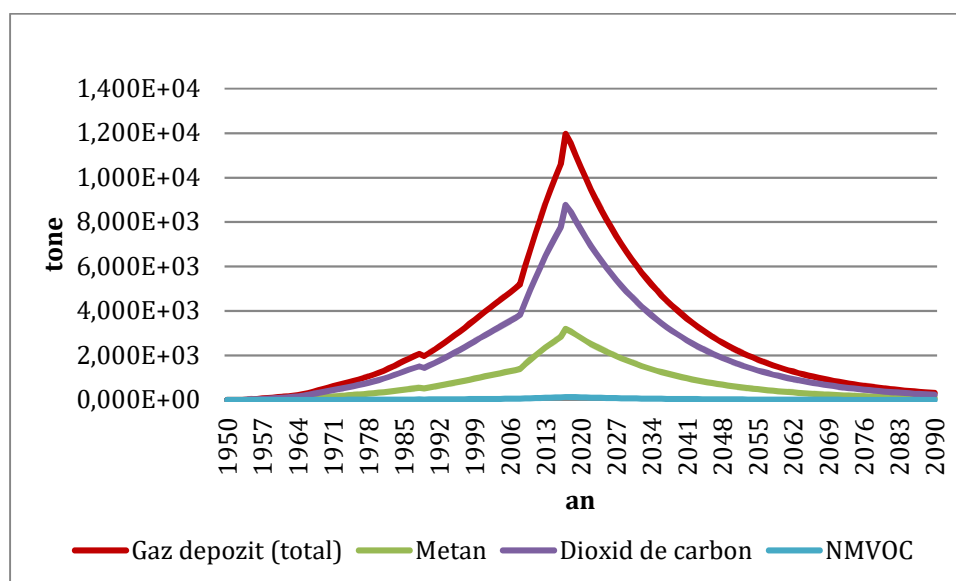
Figura 2-28: Evoluția în timp (estimativă) a emisiilor de gaze de depozit (exprimată în tone/an) pentru perioada 2021-2161 – depozit neconform Tecuci
