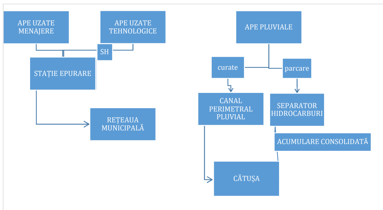
Figura 2-22: Traseul apelor evacuate în cadrul TMB
