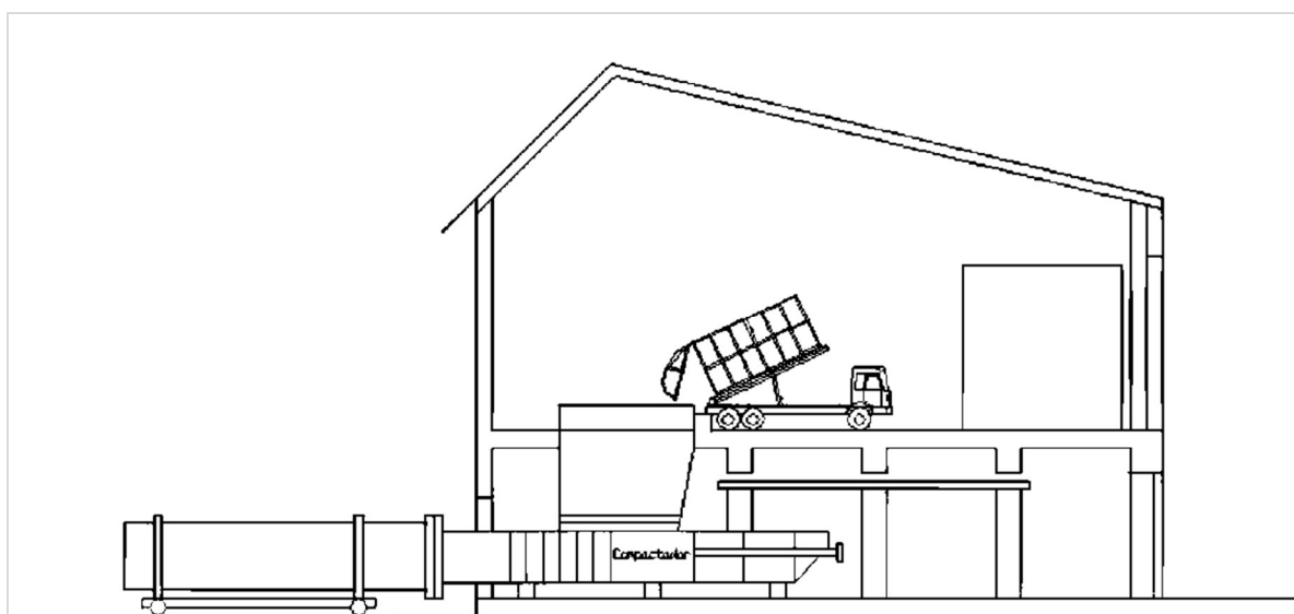
Figura 4-3: Exemplu stații de transfer cu compactare
