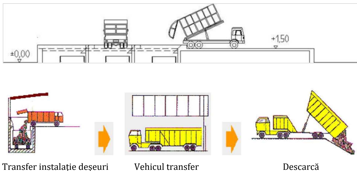
Figura 4-2: Exemplu stație de transfer fără compactare
