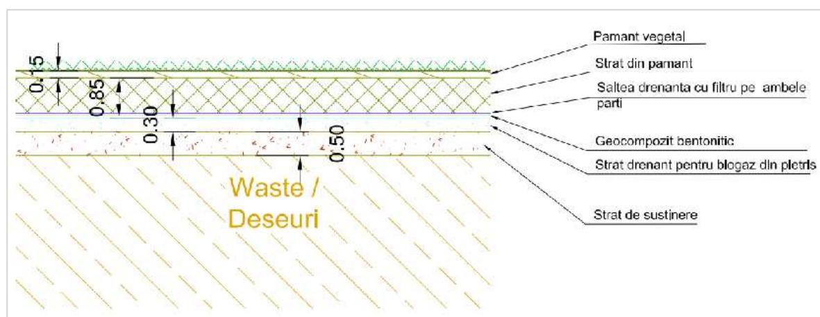
Figura 2-9: Structura sistemului de impermeabilizare
