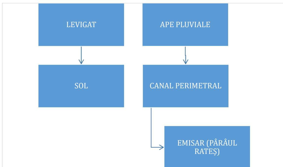
Figura 2-25: Traseul apelor evacuate și a levigatului în cadrul închiderii depozitului neconform Tecuci
