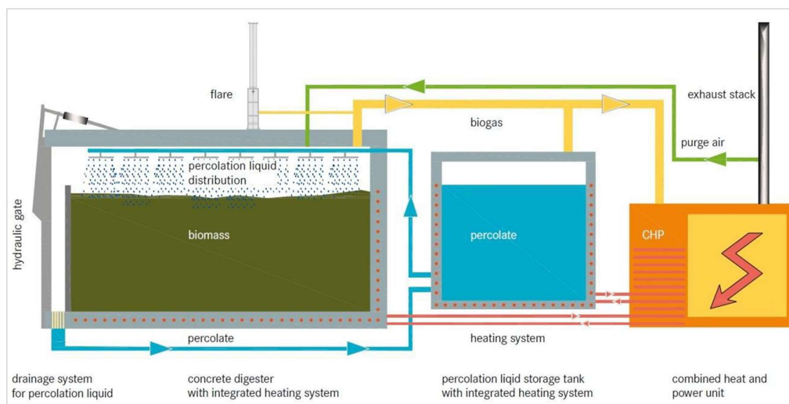
Figura 2-14: Exemplu sistem de extragere, stocare, tratare și ardere a gazului
