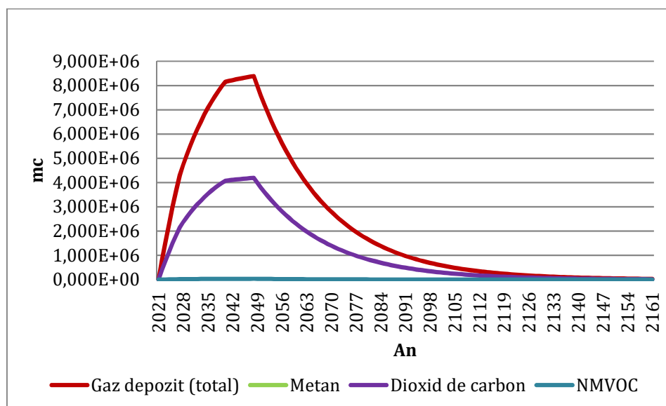
Figura 2-27: Evoluția în timp (estimativă) a emisiilor de gaze de depozit (exprimată în mc/an) pentru perioada 2021-2161 - depozit conform Valea Mărului
