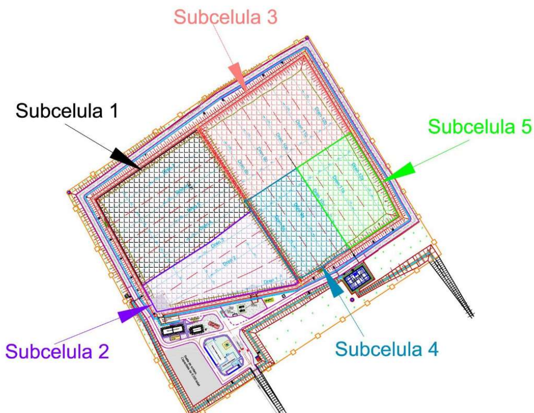
Figura 2-8: Planul de operare a depozitului Valea Mărului
