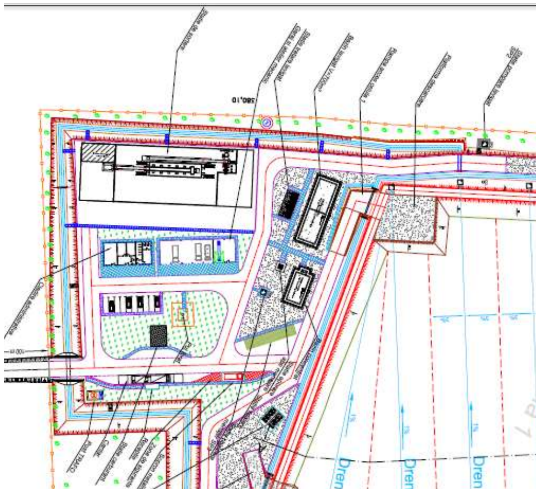
Figura 2-10: Planul general de situație stației de sortare Valea Mărului
