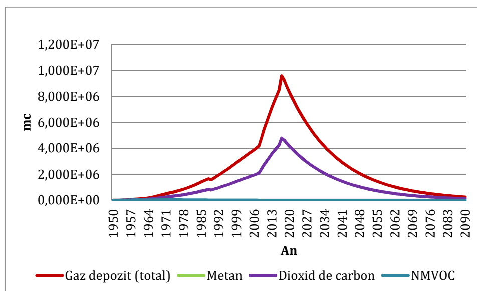
Figura 2-29: Evoluția în timp (estimativă) a emisiilor de gaze de depozit (exprimată în mc/an) pentru perioada 2021-2161 – depozit neconform Tecuci
