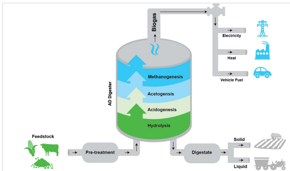
Figura 2-13: Principalele componente ale unei instalații de digestie anaerobă
