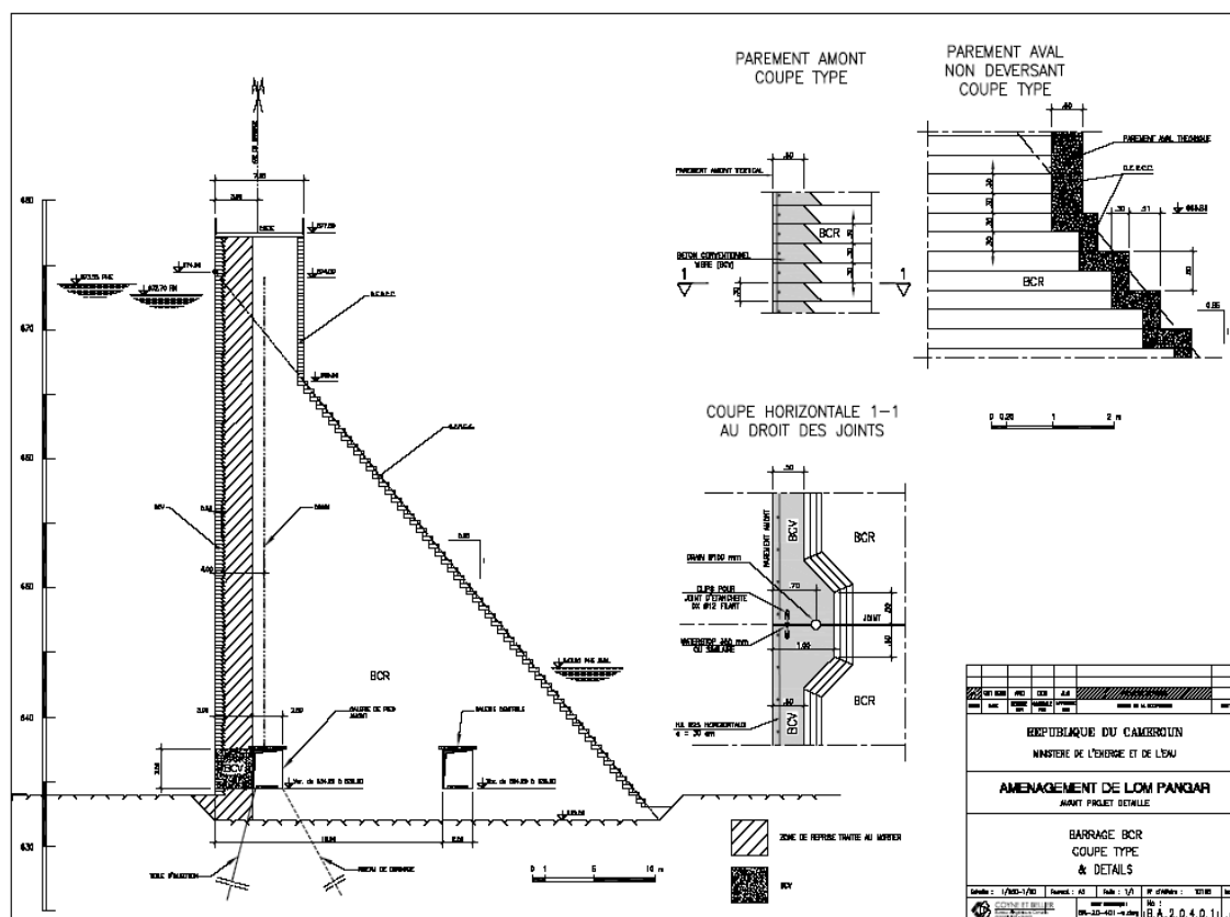
Figure 20 : Coupe type du barrage en BCR
