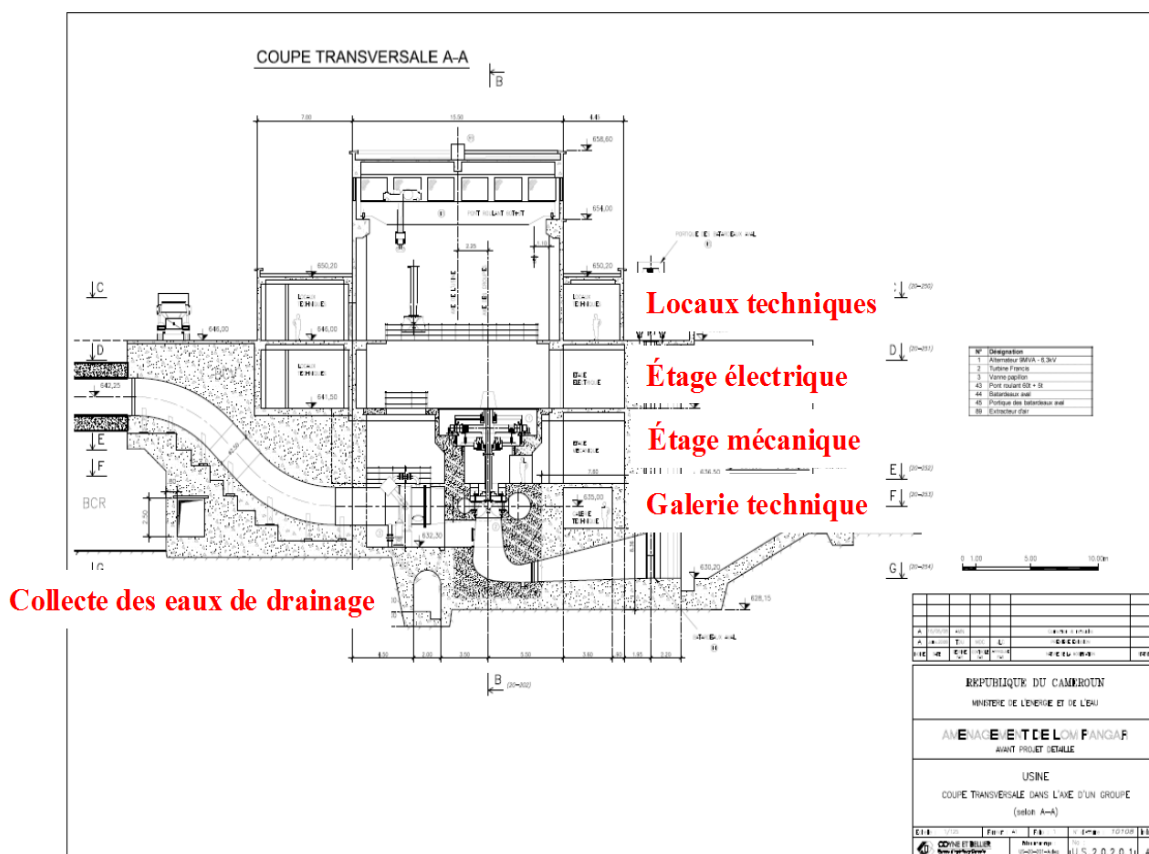
Figure 31 : Vue en coupe de l'usine
