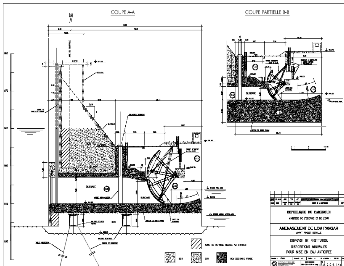
Figure 21 : Coupe sur un pertuis de fond restitution
