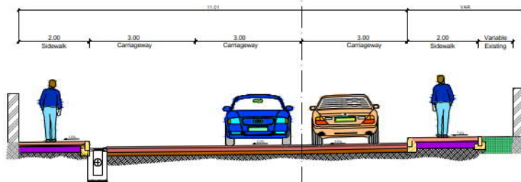
01 SECTION LAGARTO BAY (Ch 0+000 - 0+040) SCALE 1:50
