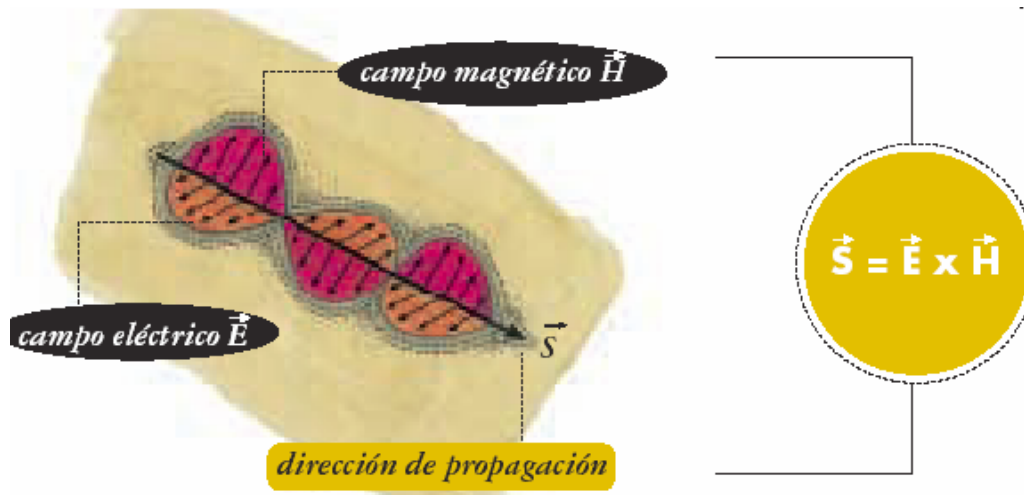
Imagen 1. Propagación de los campos eléctricos y magnéticos. Vector de Poynting.
