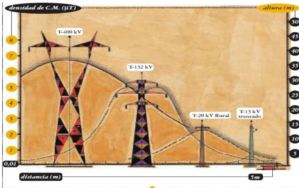
Imagen 3. Líneas eléctricas aéreas.
