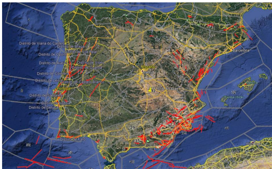
Figura 1.1.3.b. Mapa de Fallas activas cuaternarias en la Península Ibérica. Fuente:IGME.
