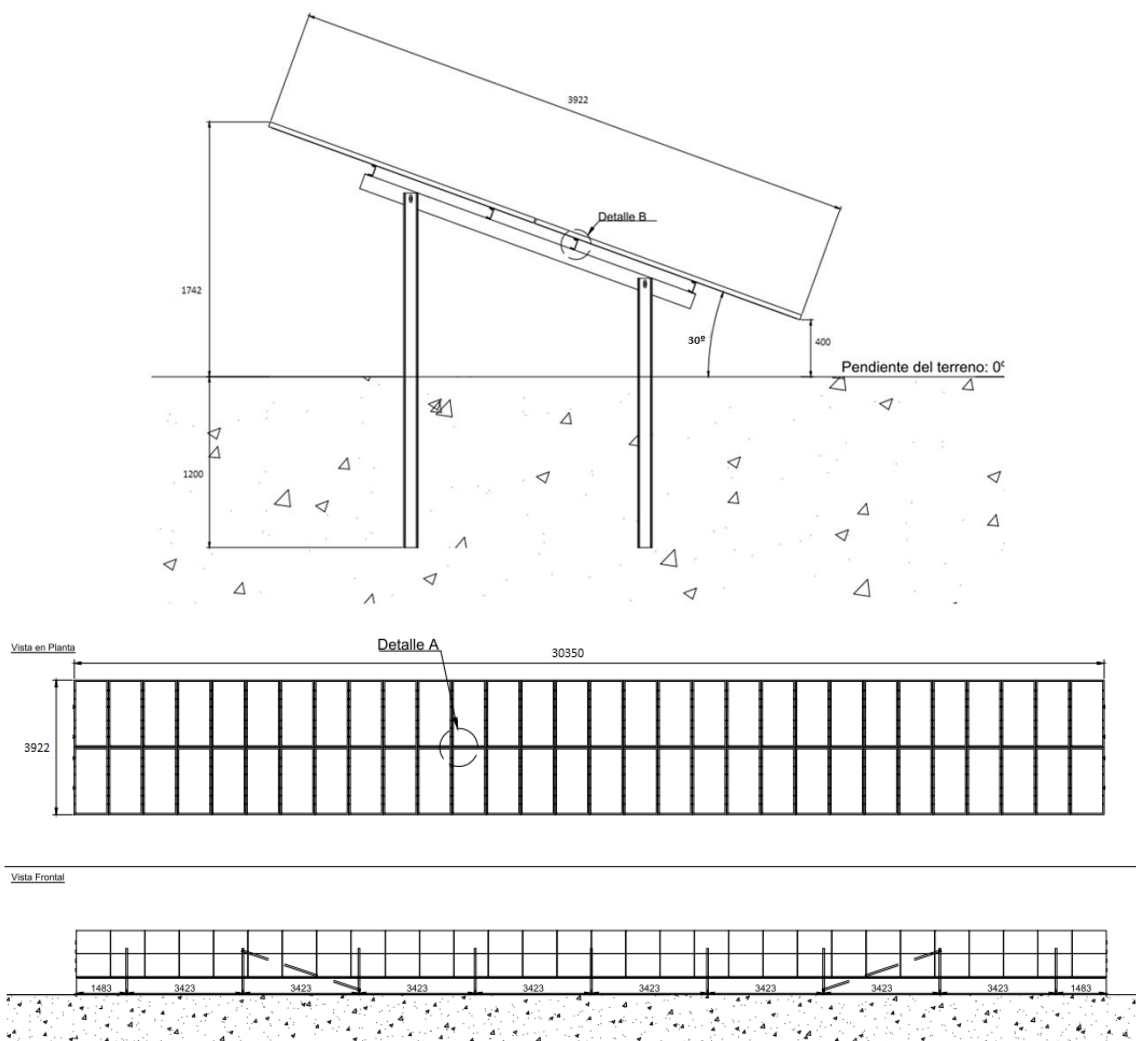
Figura 1.4.3.2.a. Vista de perfil, planta y frontal de la estructura de soporte 2Vx30. Fuente: Proyecto de Ejecución.
