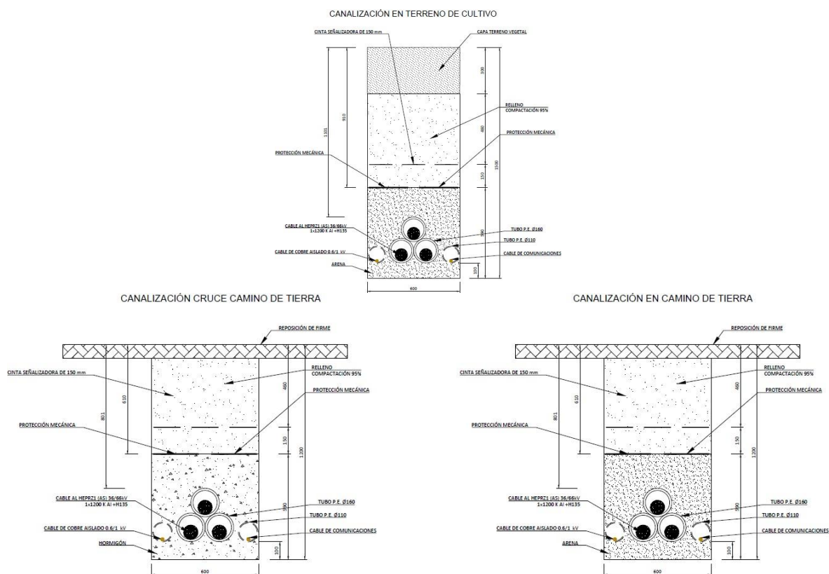
Figuras 1.6.2.a.-c. Esquema de zanjas. Fuente: Proyecto Técnico.
