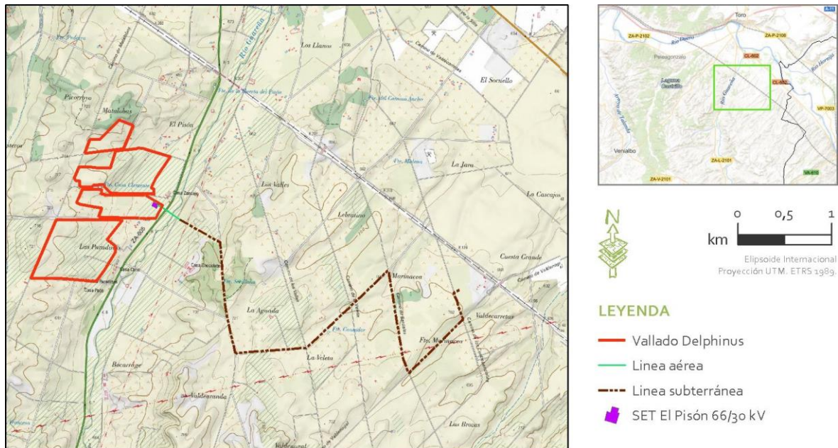
Figura 1.3.1. Localización de la PSFV Delphinus Solar 50 MW, Línea de Evacuación de 66 kV y la Subestación El Pisón 66/30 kV. Fuente: Elaboración propia.
