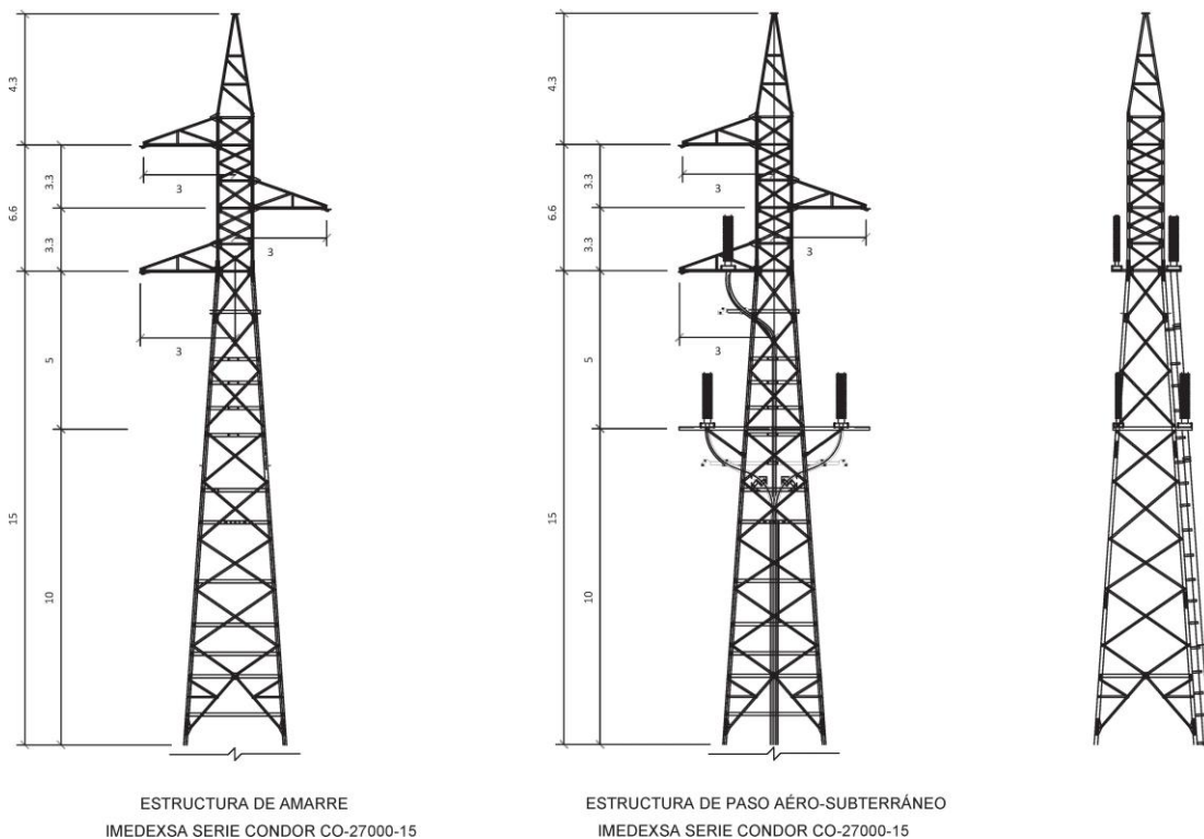
Figuras 1.6.3.a.-c. Esquema de apoyos. Fuente: Proyecto Técnico.
