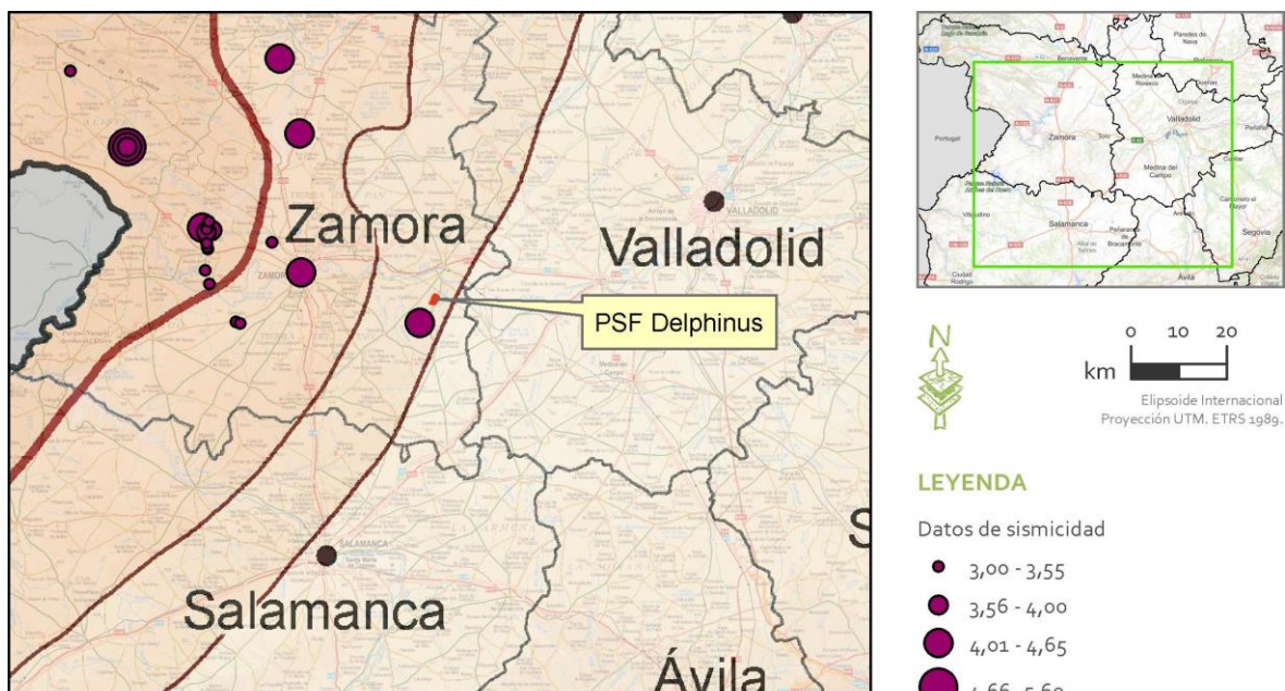
Figura 11.3.a. Peligrosidad sísmica en la zona del proyecto y registros sísmicos. Fuente: CNIG e IGME
