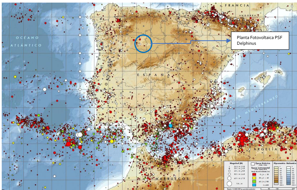
Figura 2.10.3.b. Mapa de sismicidad de la Península Ibérica (2013). Fuente: IGME.
