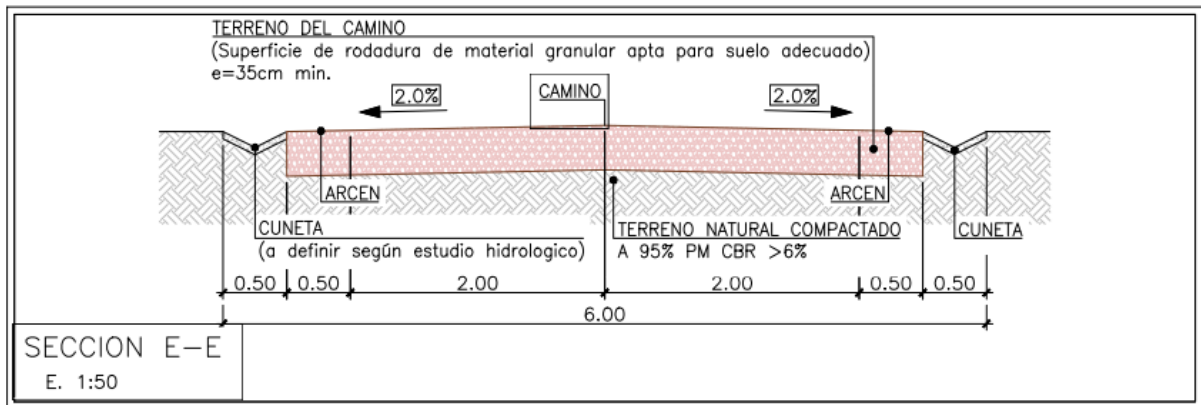
Figura 1.4.9.c. Sección tipo de viales. Fuente: Proyecto Técnico.
