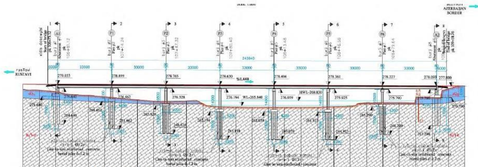
Figure 2-3. Longitudinal section
