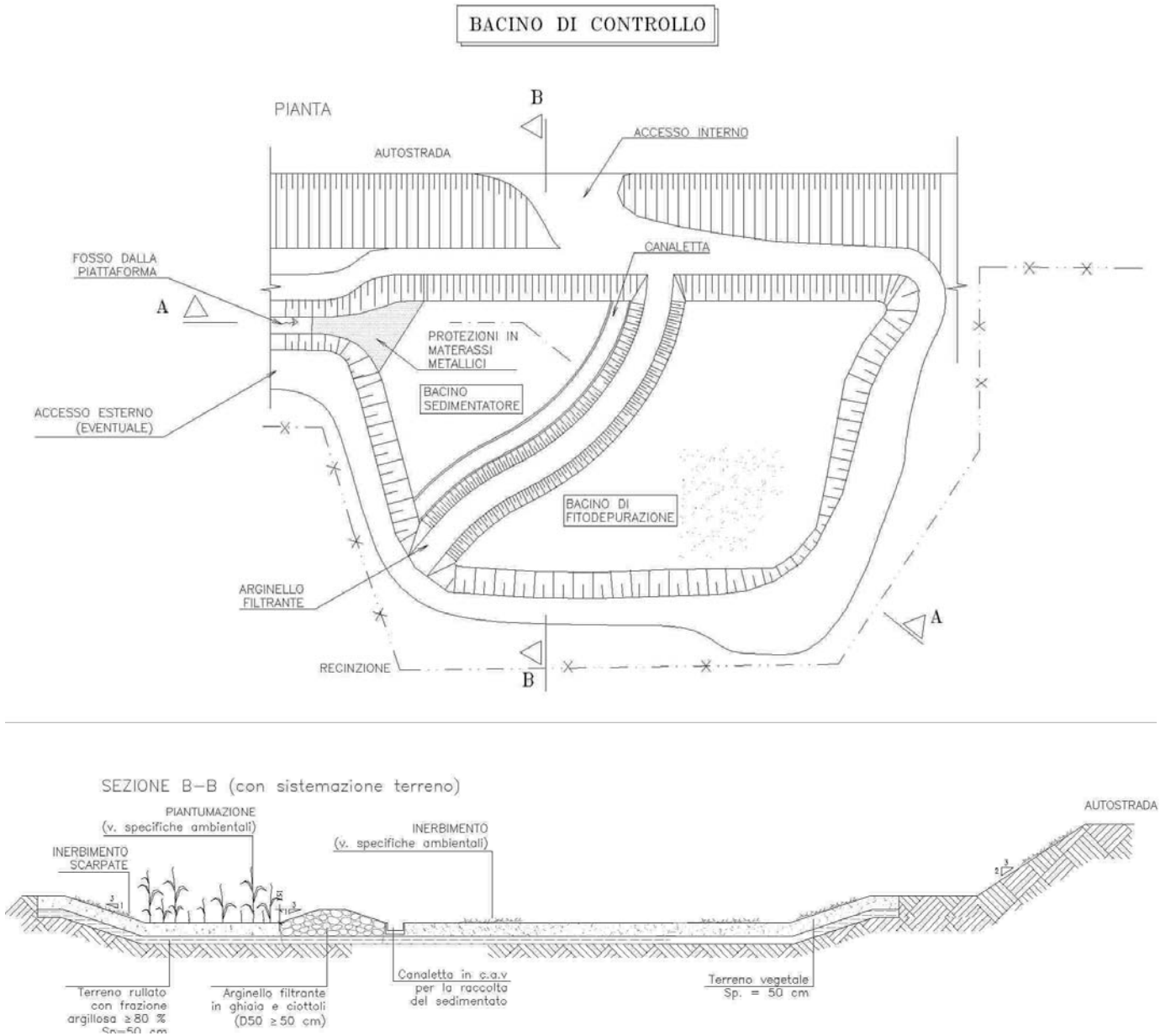
Fig. 10.1.A Bacino di controllo (vd. Progetto definitivo - Presidi idraulici – Tav. 2)
