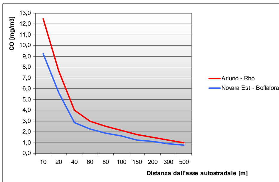
Fig. 5.4.A Andamento dei valori stimati di concentrazione del CO in relazione alla distanza dall'asse della carreggiata autostradale
