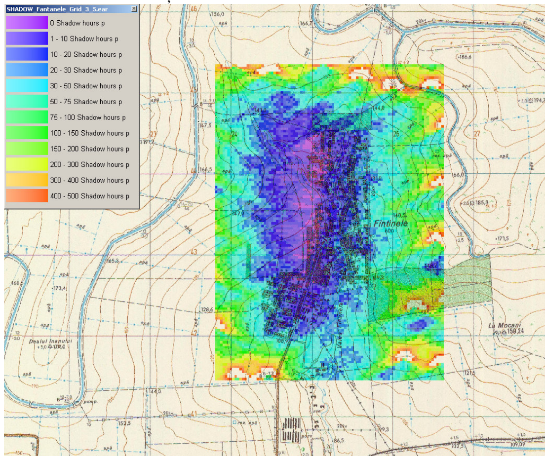
Harta cu zonele din localitatea Fantanele influentate de umbra turbinelor eoliene (ore/an)
