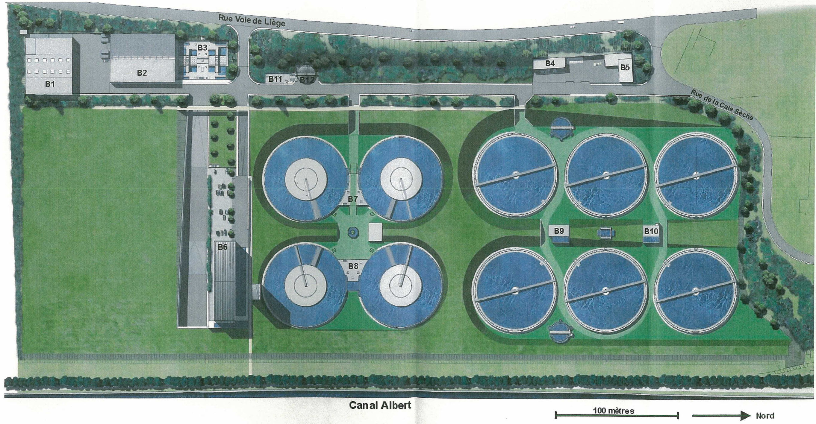
Figure 6: Plan d'implantation de la station d'épuration (source Lièg'Aqua 2002)
